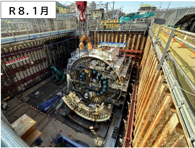
直径、長さが10mを超えるシールドマシンが組立てられていきます。
