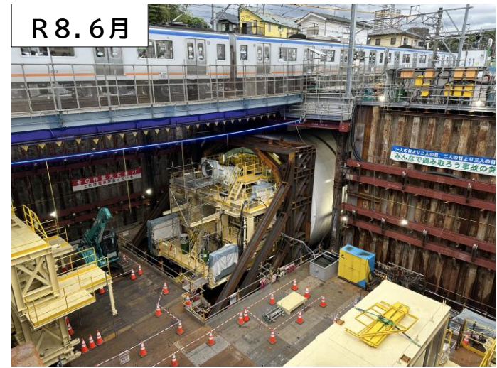
組立てた後は試運転を実施し、シールドマシンが正常に動くことを確認しました。 この後は、後ろに続く台車の接続など、付属設備の準備を行います。
