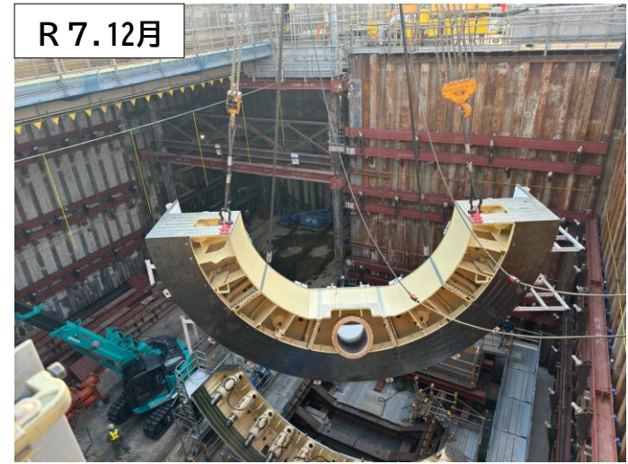
部品は最大130 tにもなります。クレーンを使い、一つずつ立坑の中に降ろしています。
